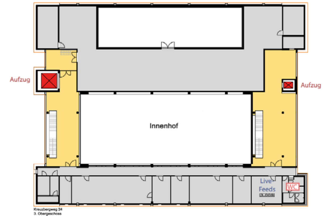
3. Obergeschoss
