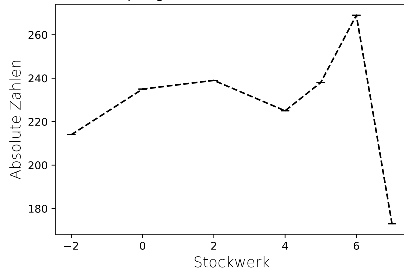
Abdämpfung durch Gebäude - Absolute Zahlen
