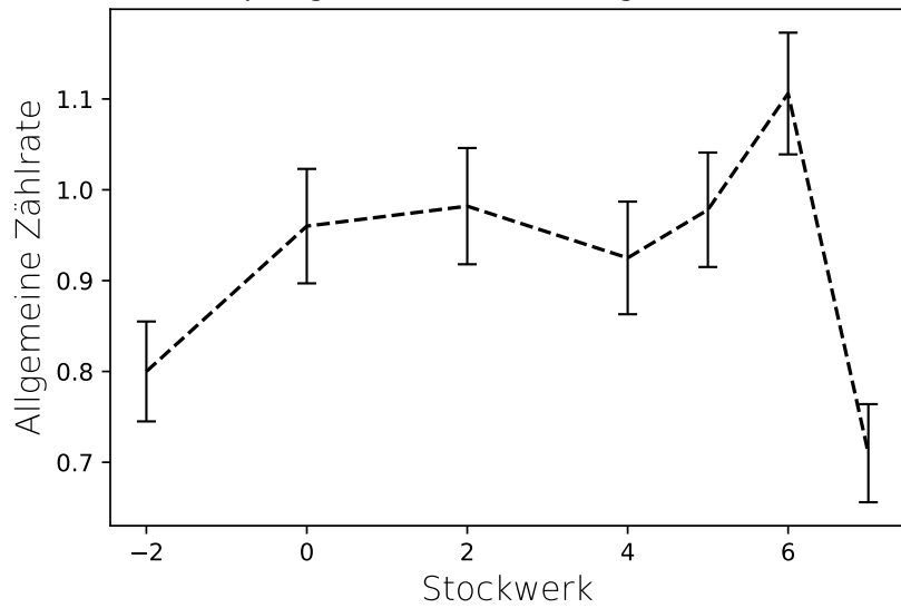
Abdämpfung durch Gebäude - Allgemeine Zählrate
