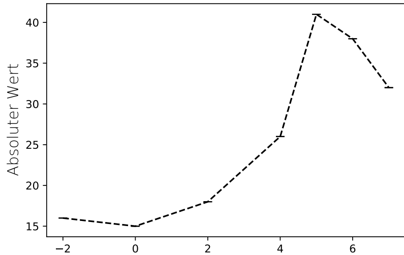
Abdämpfung durch Gebäude - totale Werte der Koinzidenzmessung
