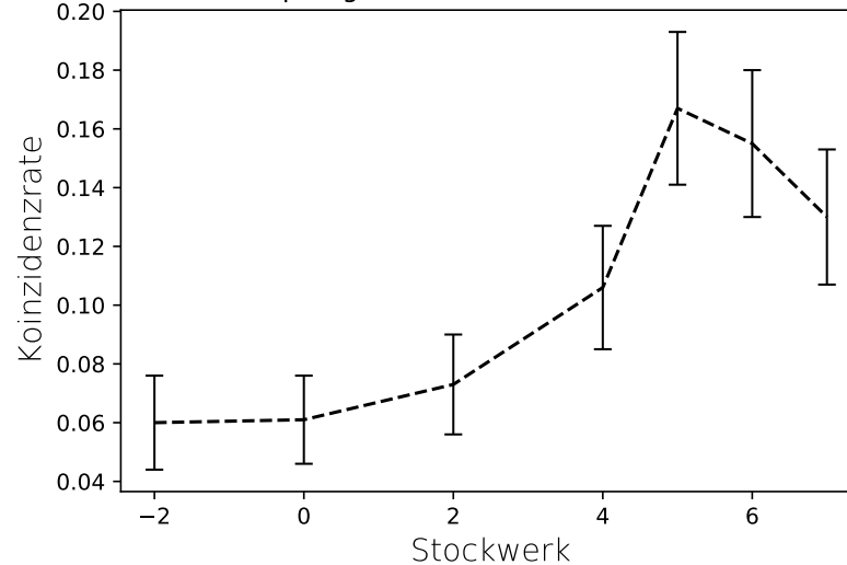
Abdämpfung durch Gebäude - Koinzidenzrate
